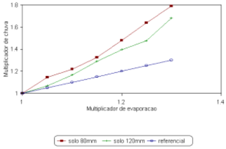
Fig. 5.2 - Região dos Inhamuns ciclo vegetativo 90 dias
