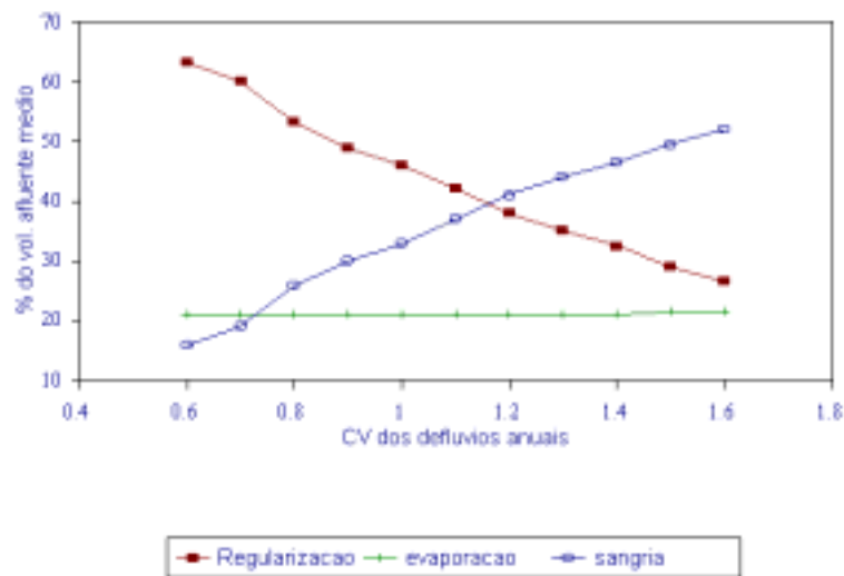
Fig. 10 Regularizacao x CV(defluvios) valores para f_k = 2,0 e f_e = 0,20
