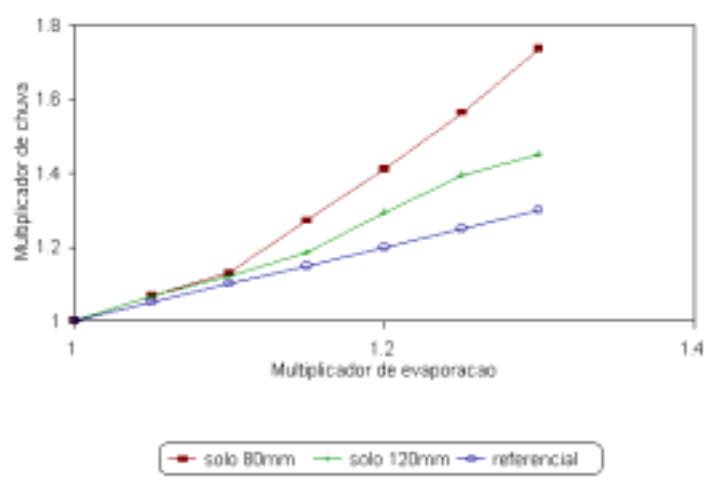
Fig. 5.3 Região do Litoral ciclo vegetativo 90 dias
