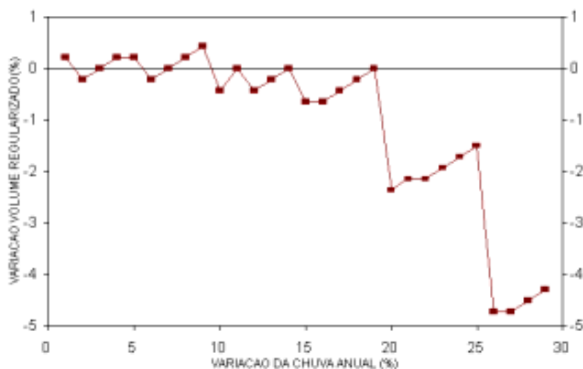
Fig 5.6 RENDIMENTO DE UM AÇUDE CENÁRIO DE MUDANÇAS CLIMÁTICAS
