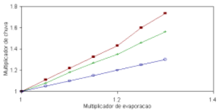
Fig. 5.2 - Região dos Inhamuns ciclo vegetativo 90 dias
