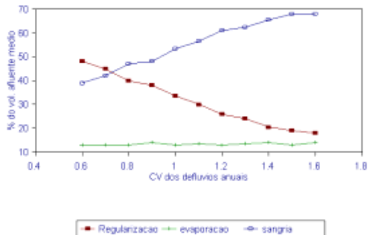
Fig 5.5 Regularizacao x CV(defluvios) valores para f_k = 1,0 ; f_e = 0,20
