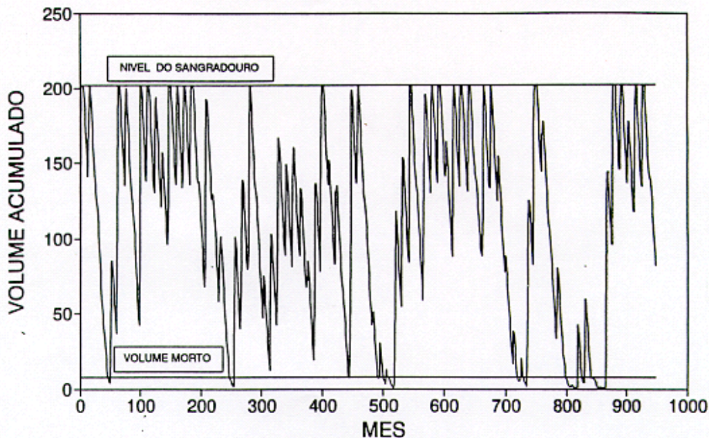
Fig. 4.2 Operação simulada do Caxitore Retirada 66 hm 3 /ano; Garantia 90% mensal
