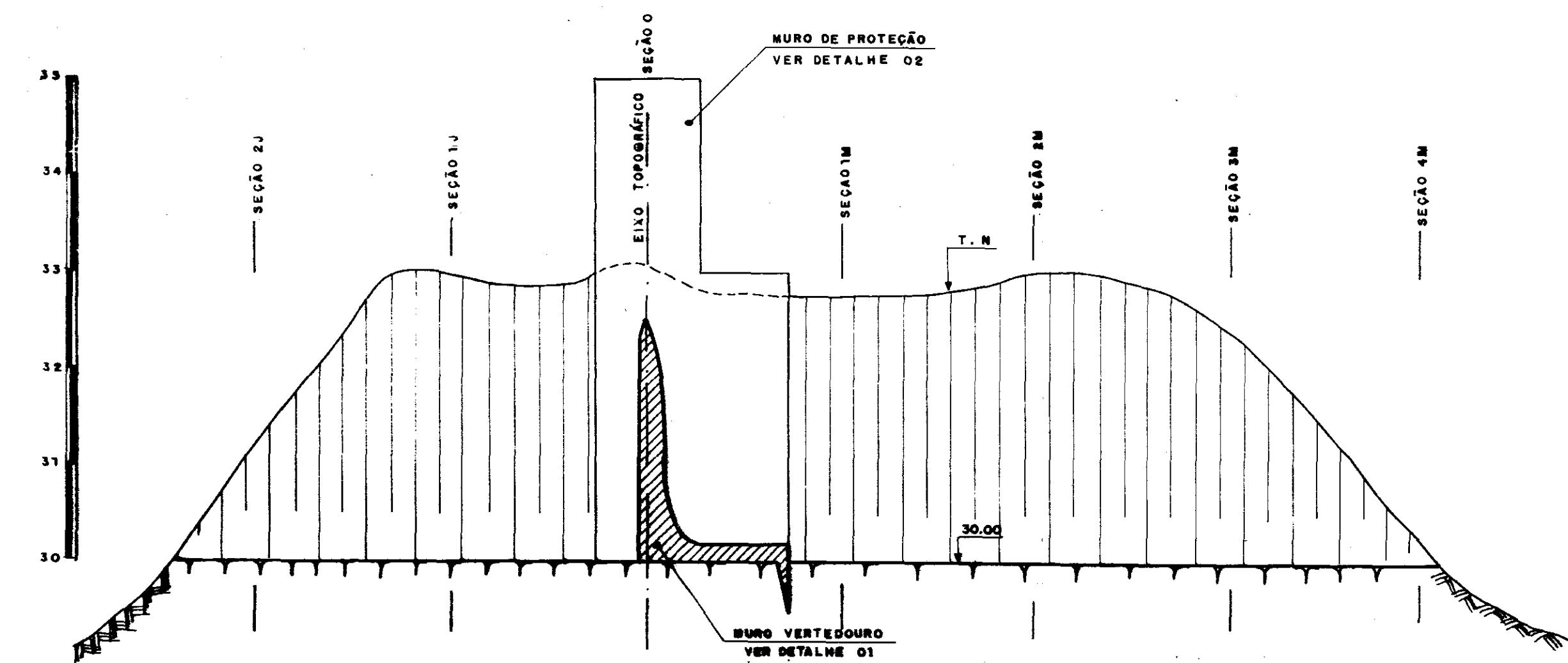
SEÇÃO LONGITUDINAL H - 1:500 ESCALAS V - 1:50
