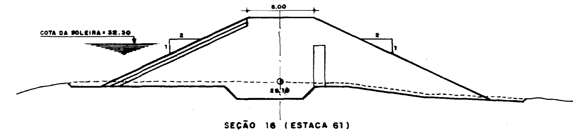
SEÇÃO 16 (ESTACA 61)
