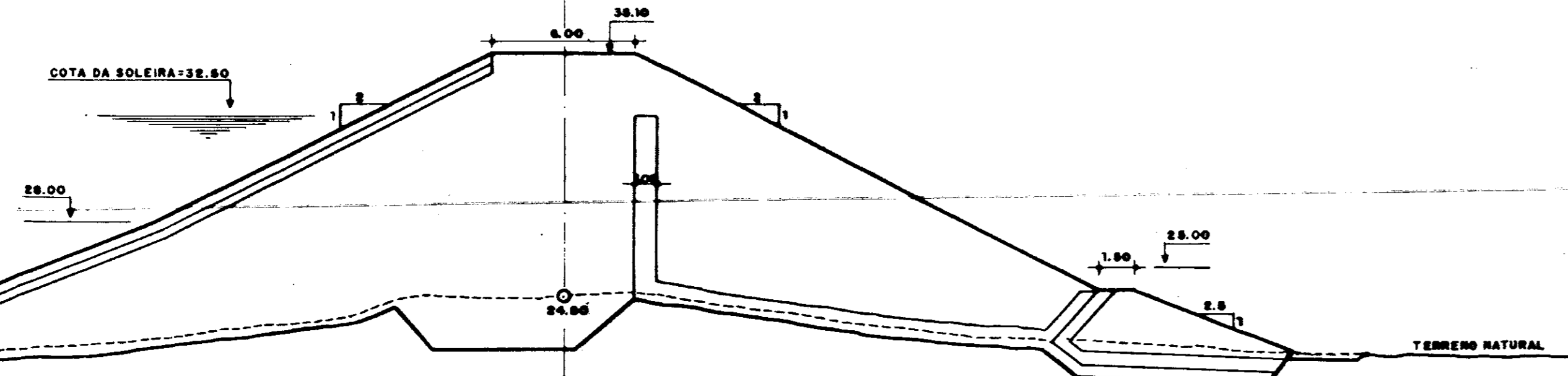
SEÇÃO 03 (ESTACA 48)
