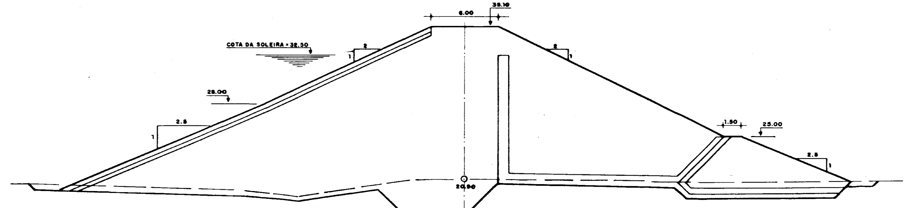
SEÇÃO 07 (ESTACA 52)
