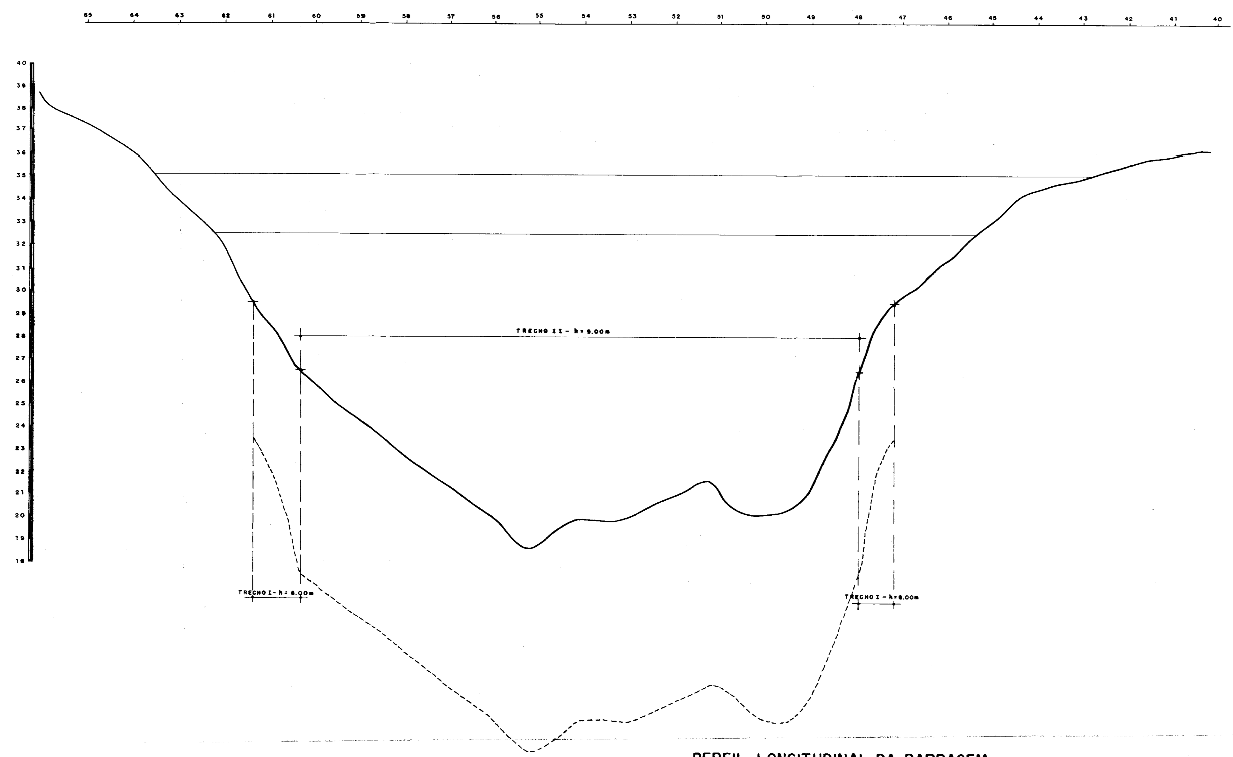
PERFIL LONGITUDINAL DA BARRAGEM
