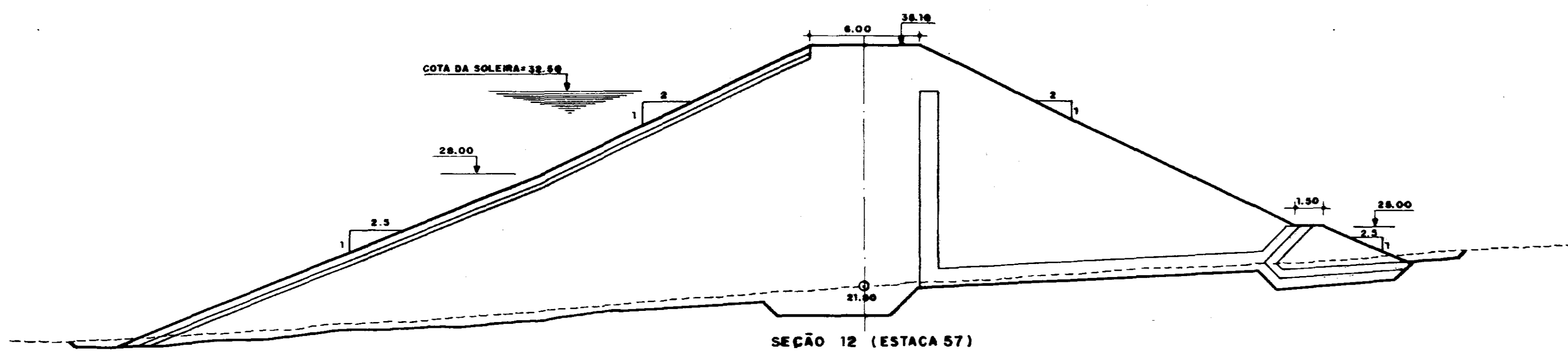
SEÇÃO 12 (ESTACA 57)
