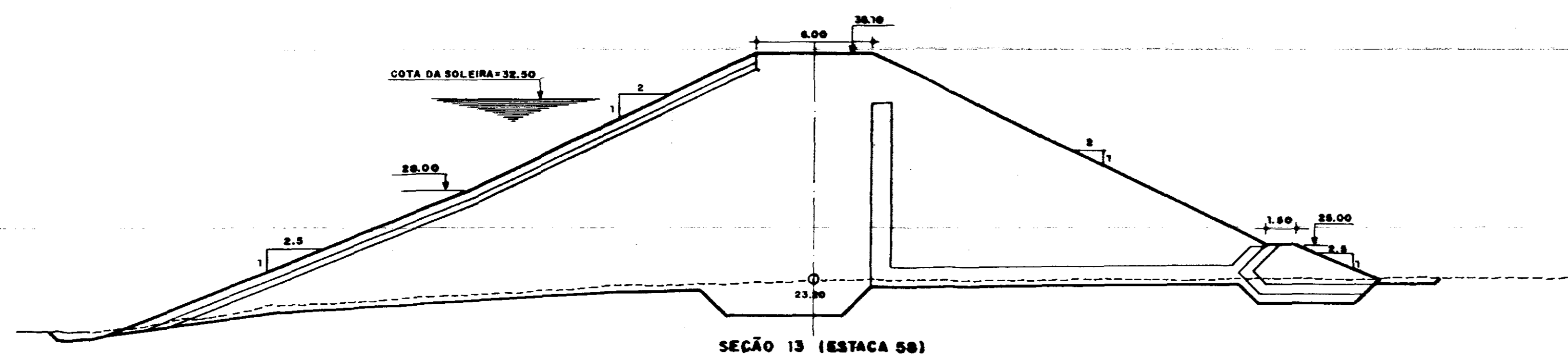
SEÇÃO 13 (ESTACA 58)
