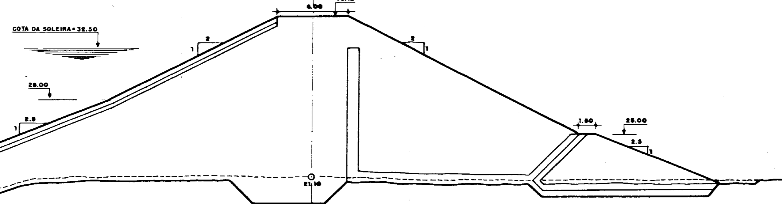
SEÇÃO 04 (ESTACA 49)
