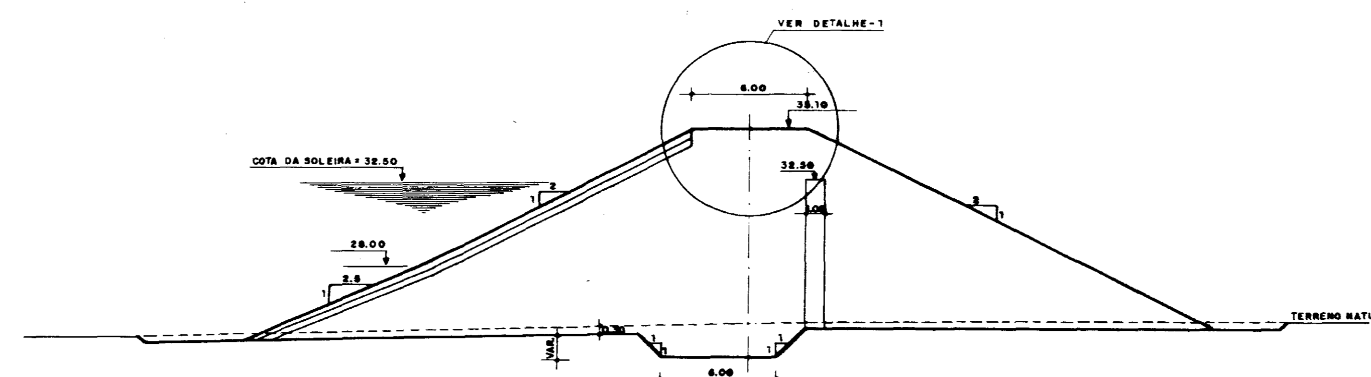
SEÇÃO TIPO (TRECHO OMBREIRAS)
