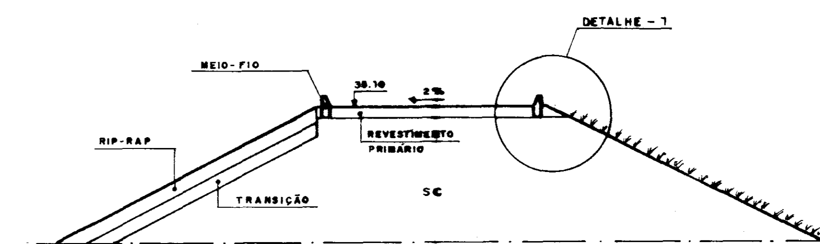
DETALHE DA CRISTA
