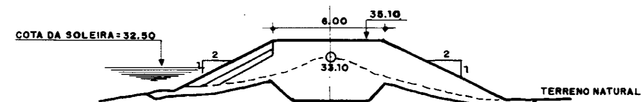
SEÇÃO 00 (ESTACA 45)
