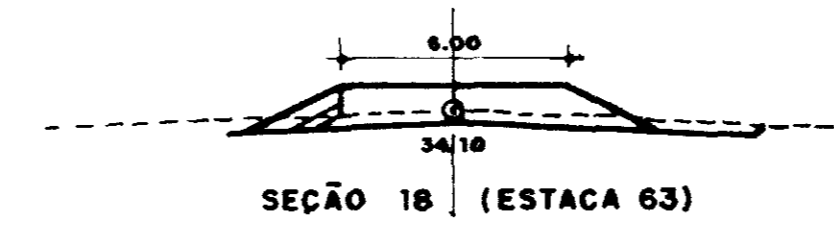
SEÇÃO 18 (ESTACA 63)
