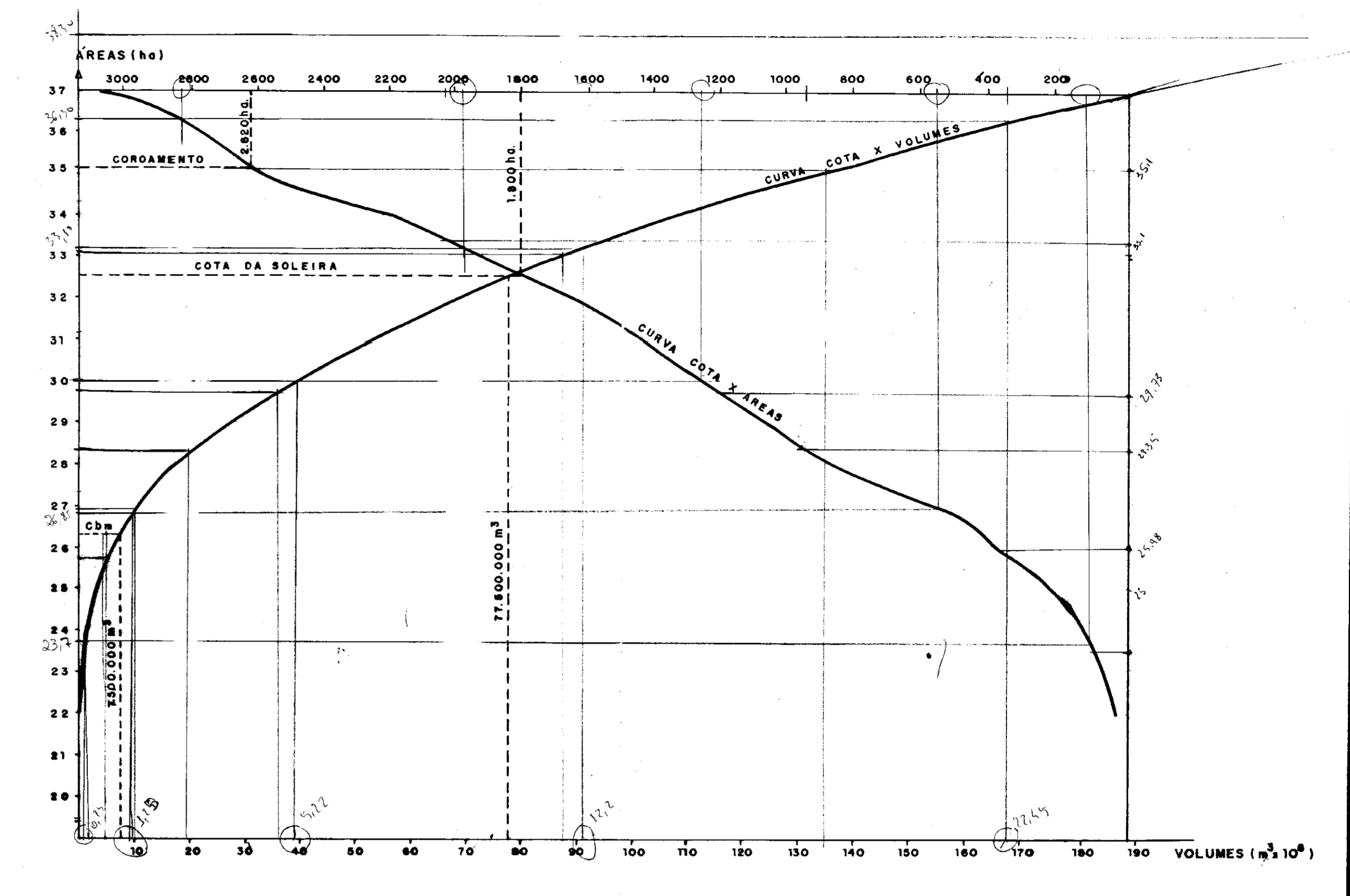
DIAGRAMA COTAS x ÁREAS x VOLUMES
