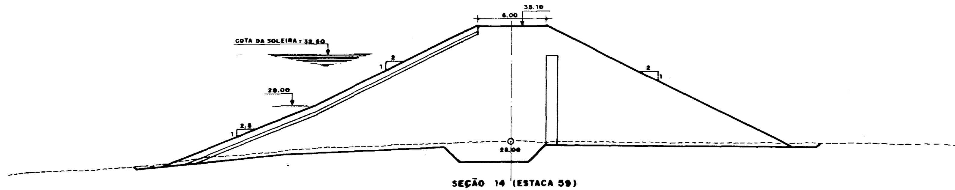
SEÇÃO 14 (ESTACA 59)
