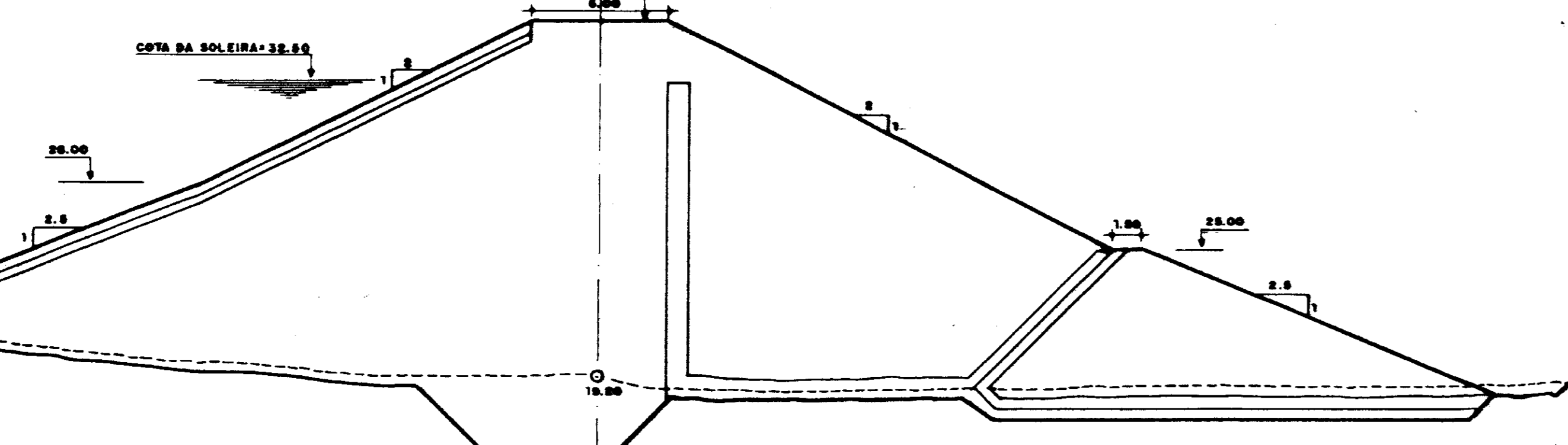
SEÇÃO 05 (ESTACA 50)
