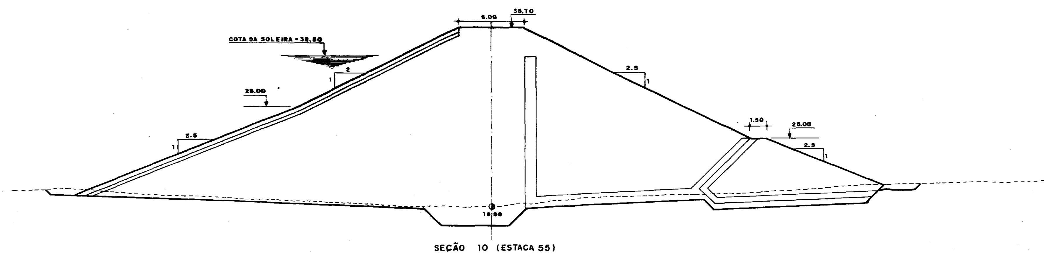
SEÇÃO 10 (ESTACA 55)
