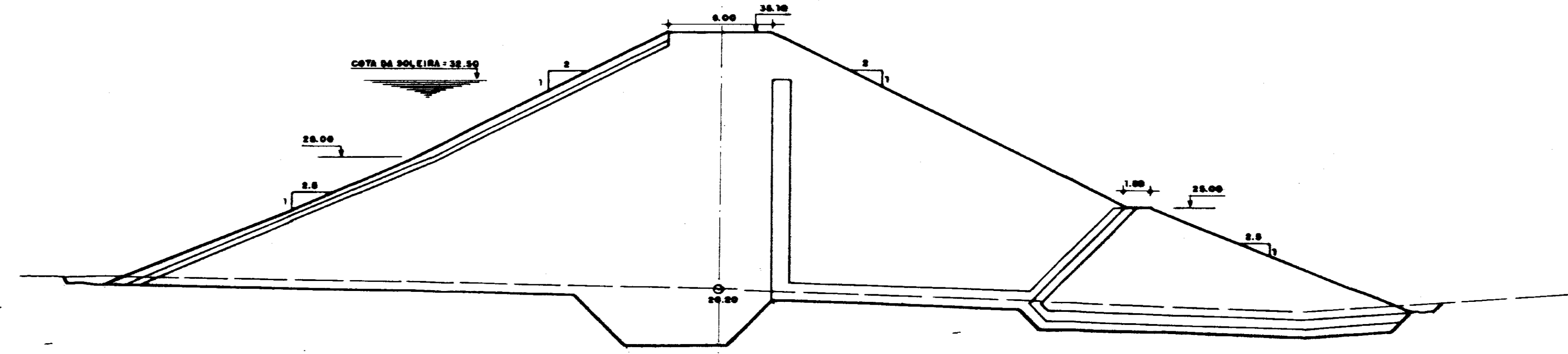
SEÇÃO 09 (ESTACA 54)
