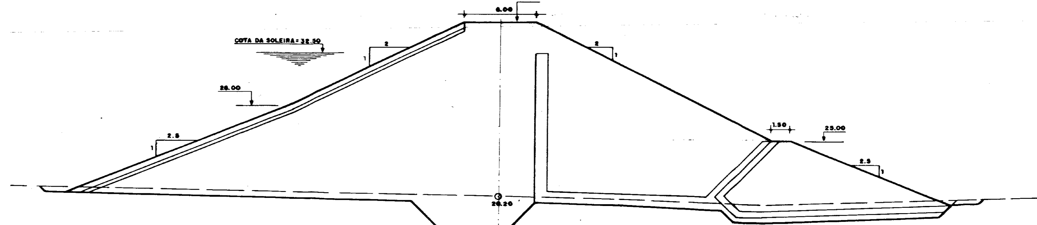
SEÇÃO 08 (ESTACA 53)
