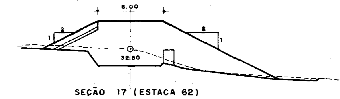
SEÇÃO 17 (ESTACA 62)
