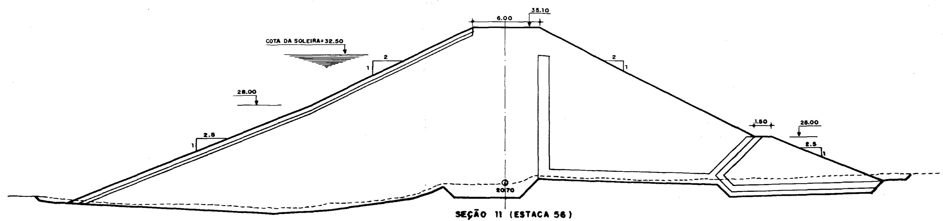
SEÇÃO 11 (ESTACA 56)
