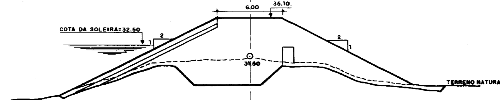
SEÇÃO 01 (ESTACA 46)
