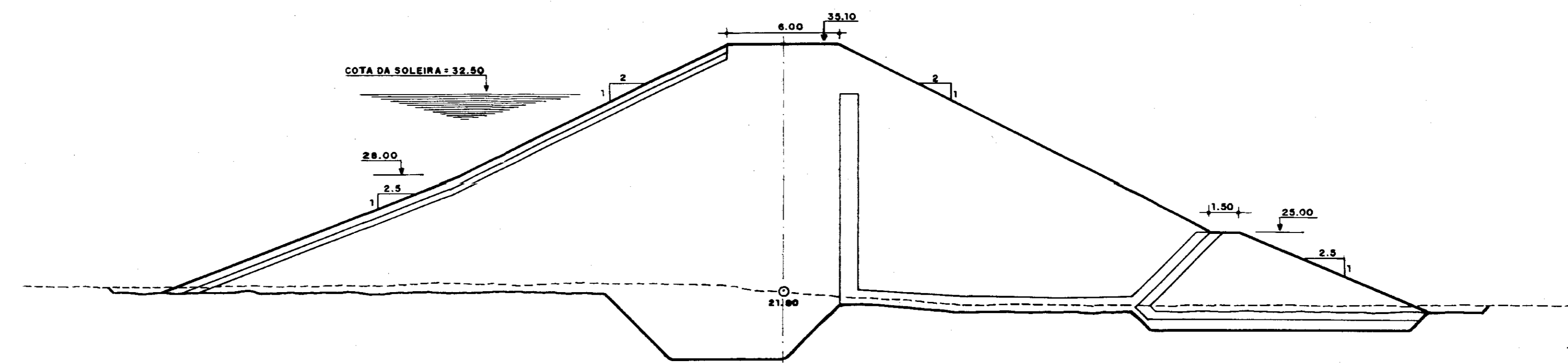
SEÇÃO 06 (ESTACA 51)
