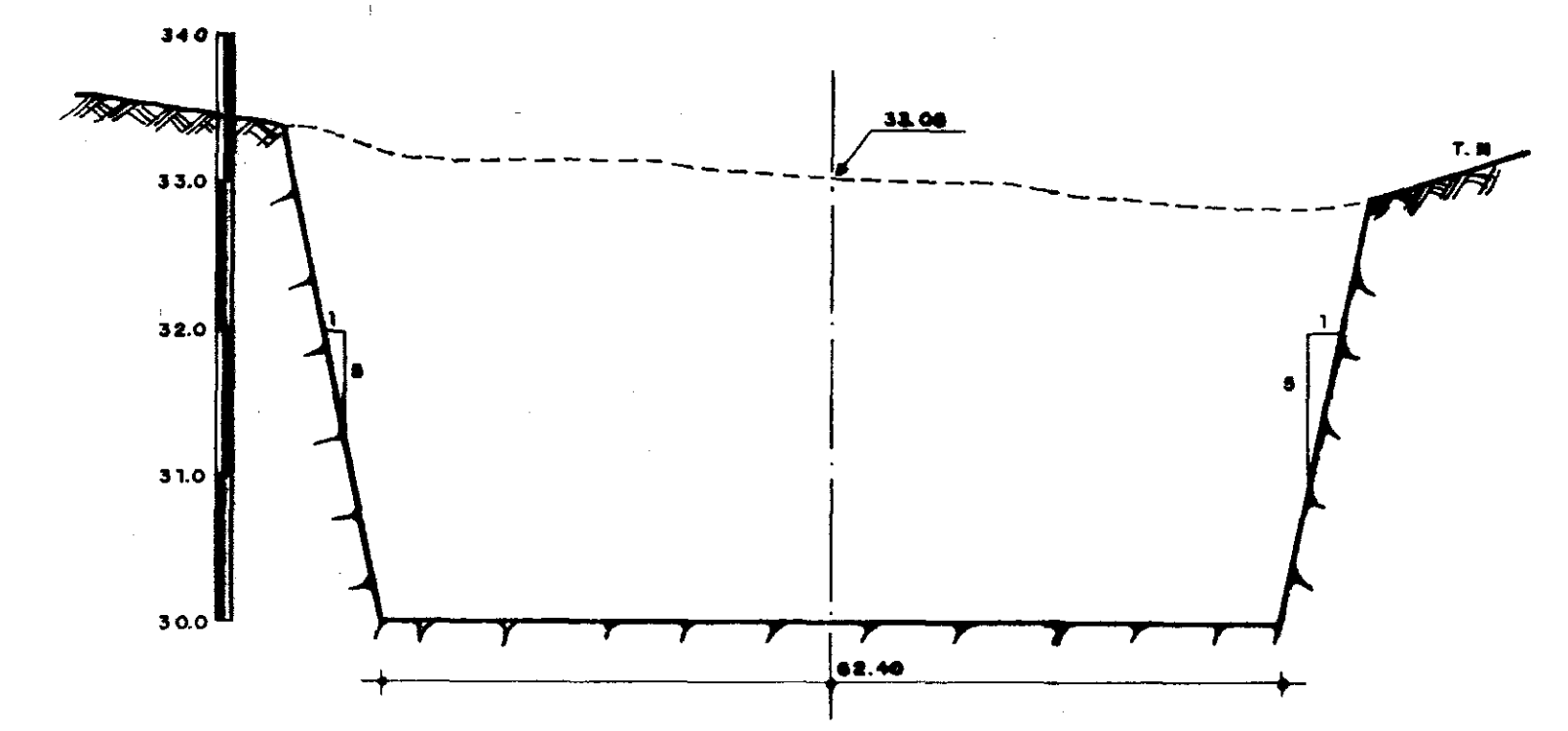
SEÇÃO 1J
