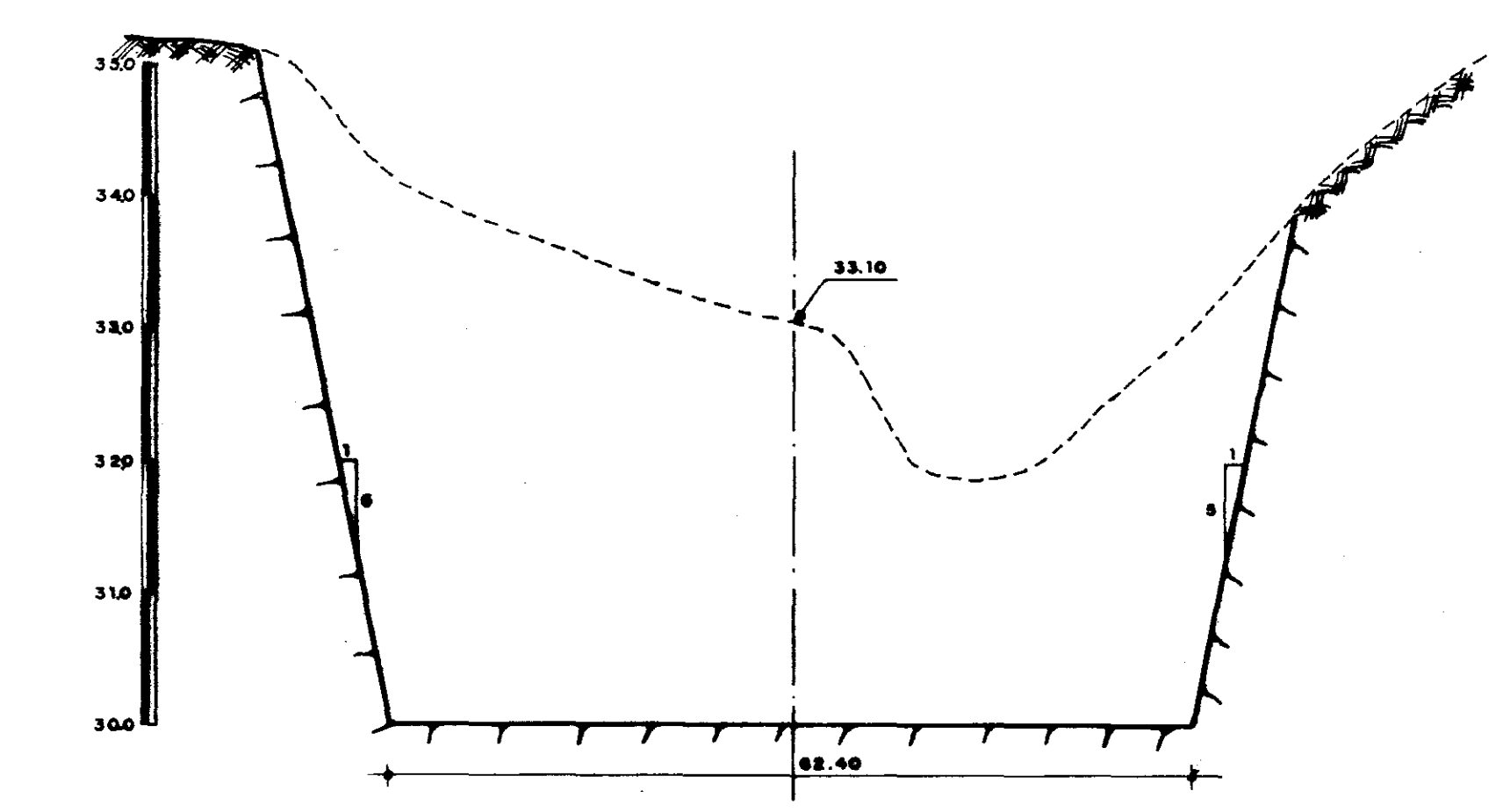
SEÇÃO 1M
