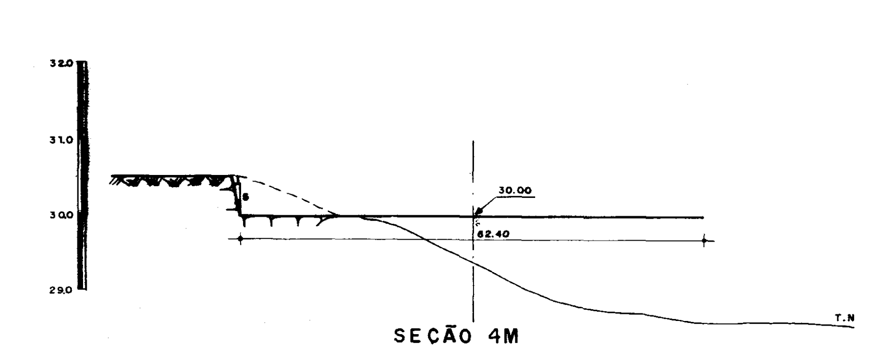
SEÇÃO 4M
