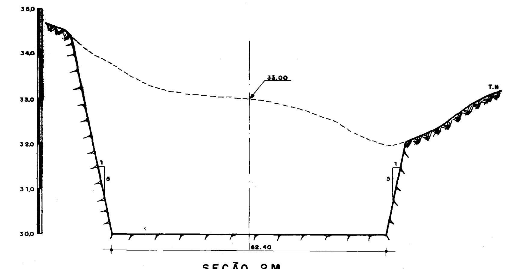
SEÇÃO 2M
