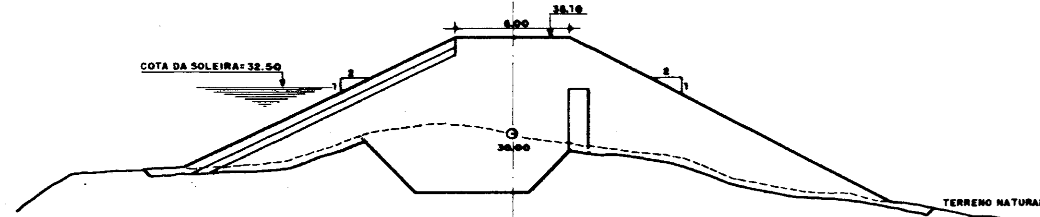
SEÇÃO 02 (ESTACA 47)
