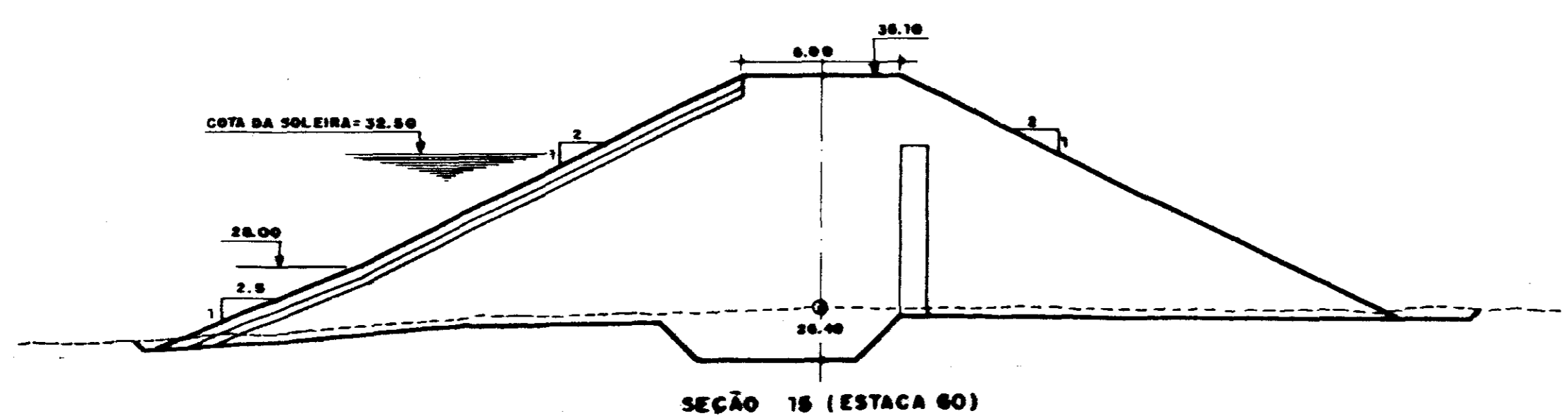
SEÇÃO 16 (ESTACA 60)
