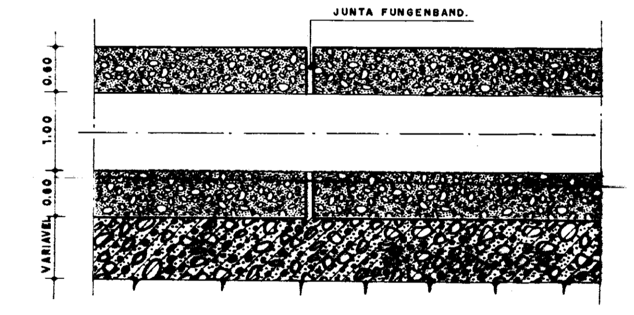
DETALHE -1 (JUNTAS) ESCALA 1:50
