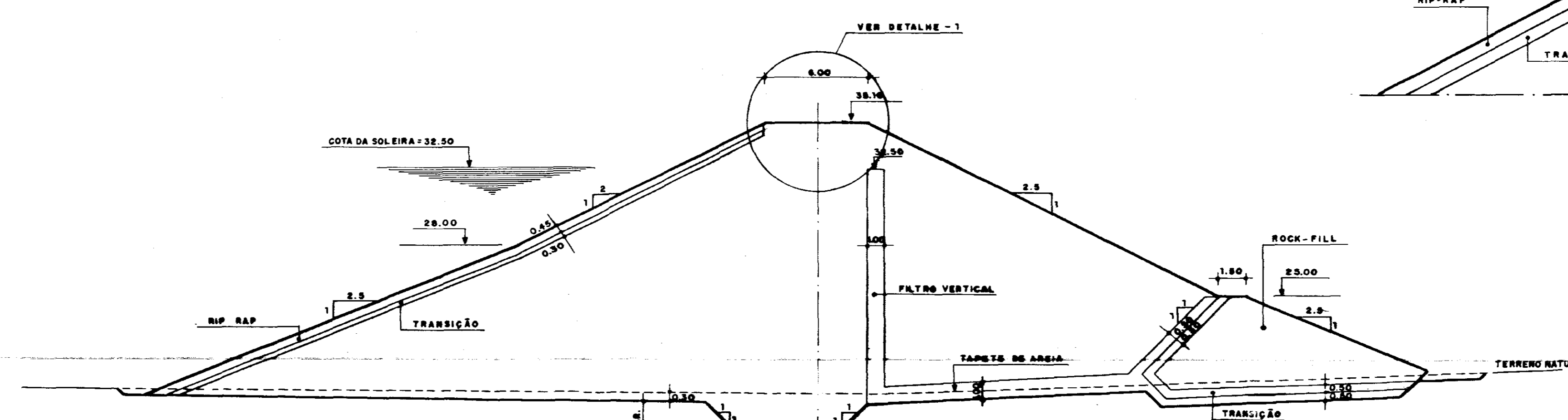
SEÇÃO TIPO (TRECHO CENTRAL)
