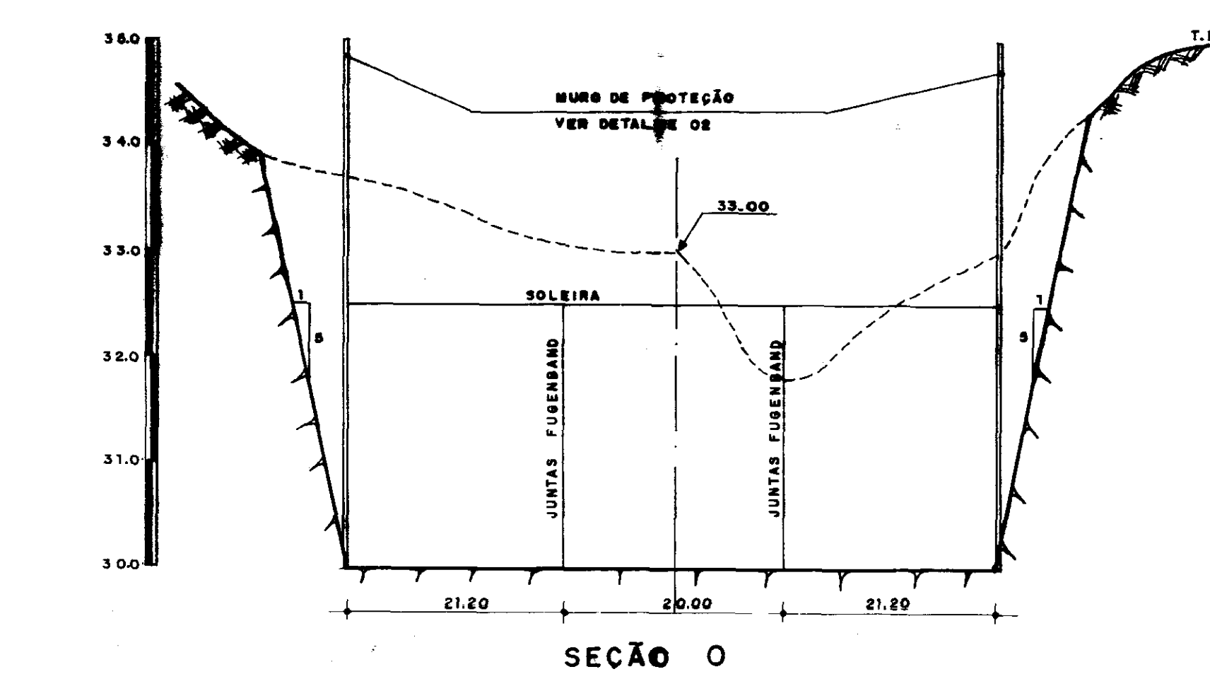
SEÇÃO 0
