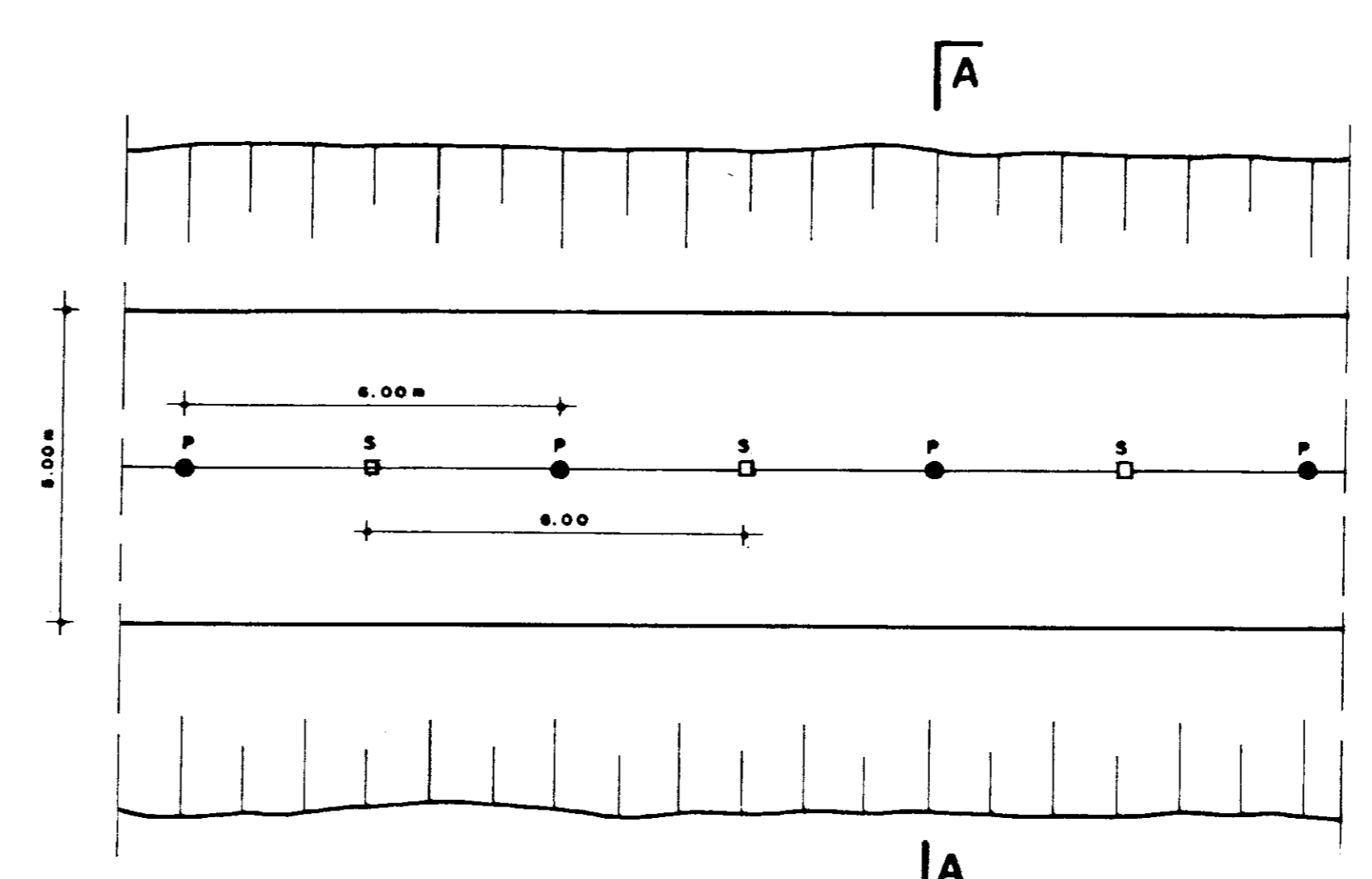
DETALHE 01 - LINHA DE INJEÇÃO
