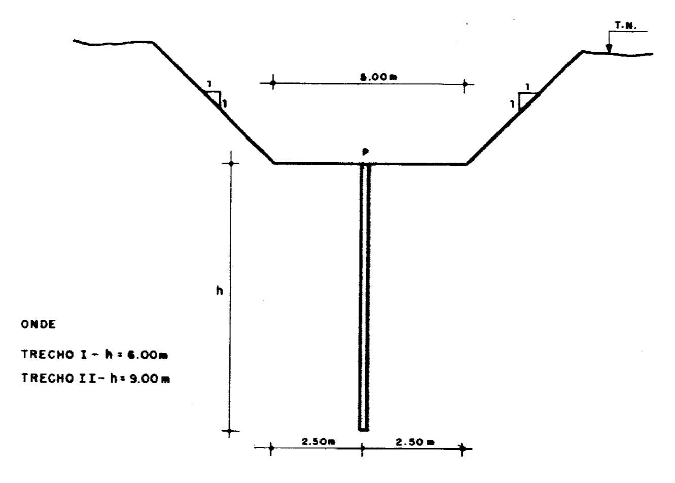
CORTE AA
