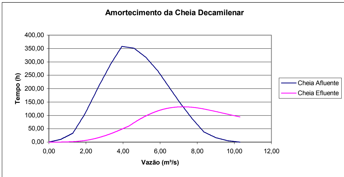
FIGURA 8.2 – Amortecimento da cheia decamilenar para cotas do vertedouro do Açude São Bernardo
