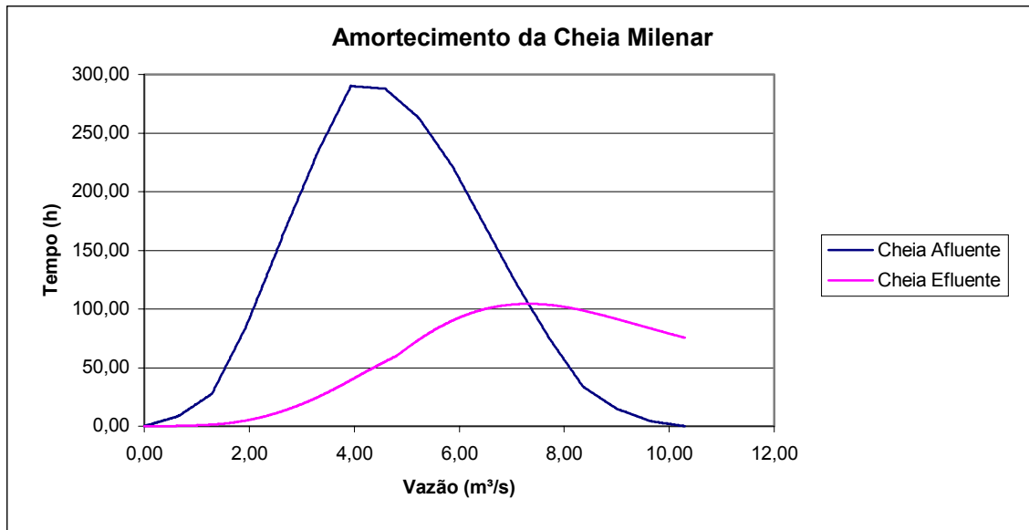
FIGURA 8.1 – Amortecimento da cheia milenar para cotas do vertedouro do Açude São Bernardo
