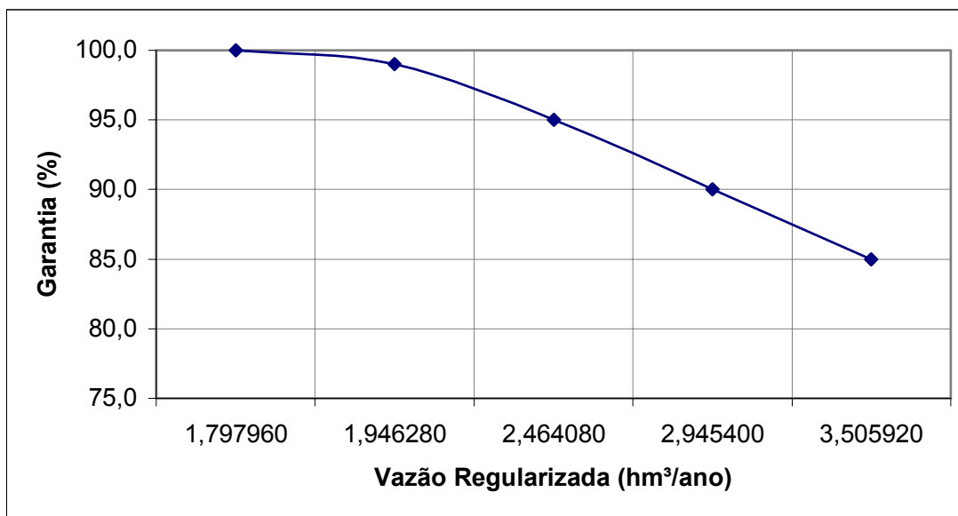
Figura 6.1 – Curva Garantia versus Vazão Regularizada do açude São Bernardo, para a Capacidade de 9,349 \text{ hm}^3 (cota = 239 m ).
