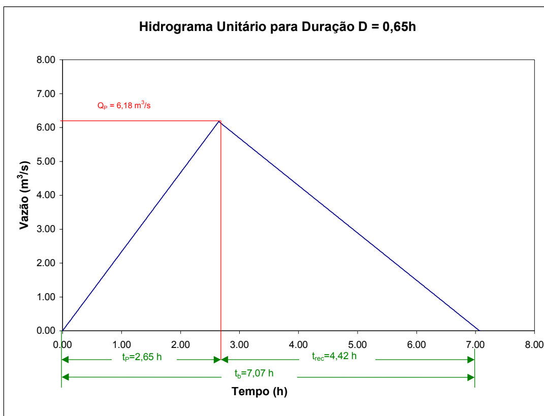
Figura 6.2 - Hidrograma unitário triangular do SCS para duração de 0,65 horas
