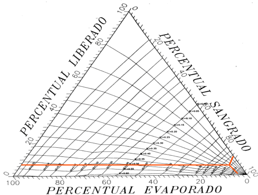
FIGURA 2.7 – DIAGRAMA TRIANGULAR DE REGULARIZAÇÃO APLICADO A BARRAGEM RIACHO DO MEIO
