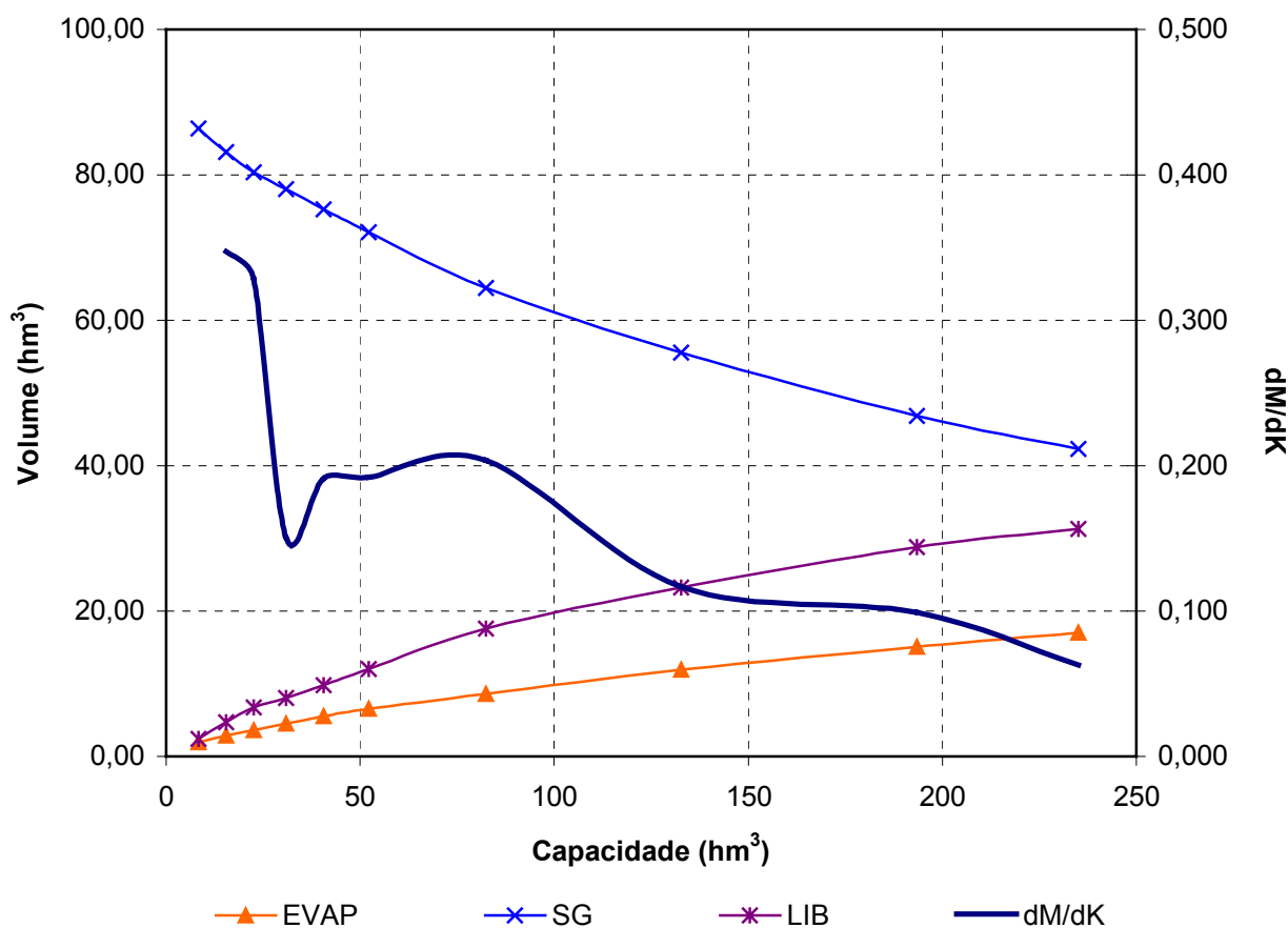
FIGURA 2.6 – CURVAS DE REGULAÇÃO DO RESERVATÓRIO RIACHO DO MEIO
