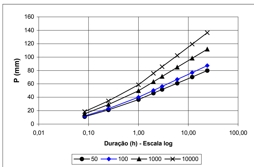
FIGURA 2.3 – CURVAS INTENSIDADE-DURAÇÃO-FREQÜÊNCIA
