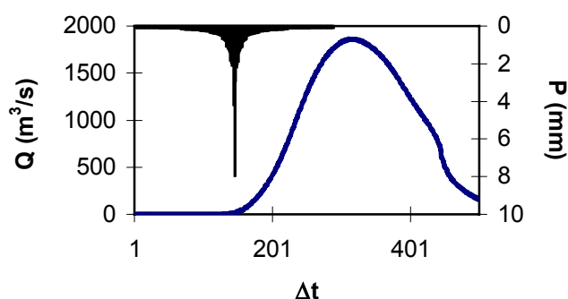
FIGURA 2.4 – HIDROGRAMA TOTAL AFLUENTE AO RIACHO DO MEIO (TR = 1000 ANOS)
