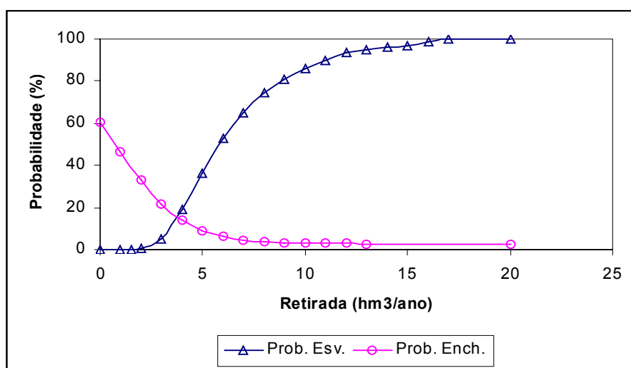
FIGURA 2.9 – PROBABILIDADES DE ESAZIAMENTO E ENCHIMENTO
