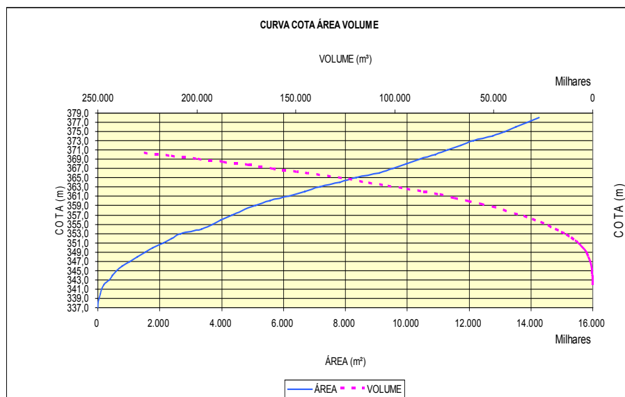
FIGURA 2.8 – CURVA COTA – ÁREA – VOLUME
