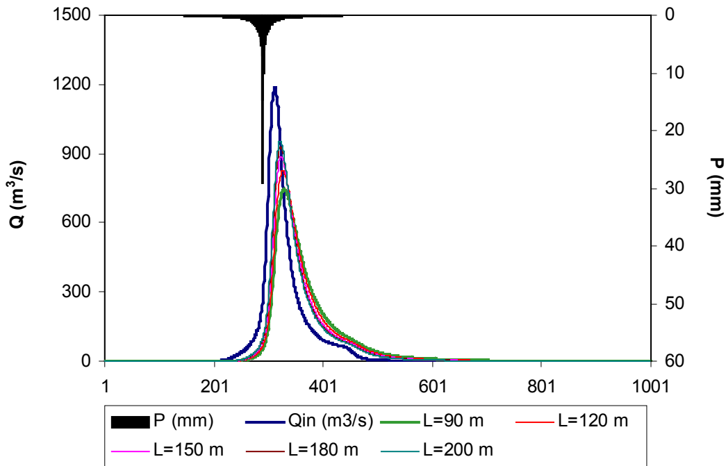
FIGURA 8.4 - HIDROGRAMAS DE ENTRADA E DE SAÍDA DO RESERVATÓRIO RIACHO DO MEIO (TR=10.000 ANOS, PERFIL CREAGER, CHUVA = 2 DIAS)
