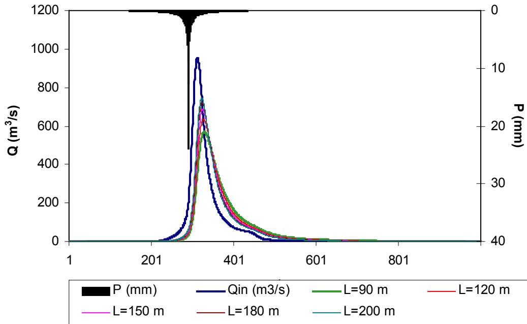
FIGURA 8.3 - HIDROGRAMAS DE ENTRADA E DE SAÍDA DO RESERVATÓRIO RIACHO DO MEIO (TR=1.000 ANOS, PERFIL CREAGER, CHUVA = 2 DIAS)
