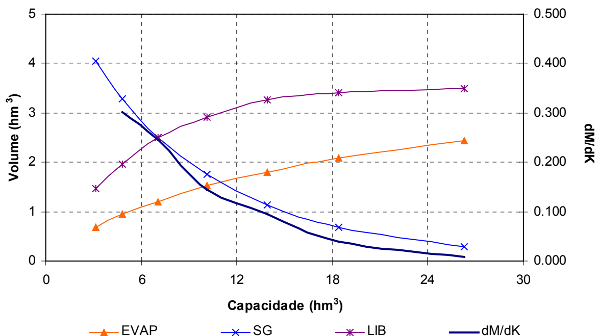
FIGURA 7.1 – CURVAS DE REGULAÇÃO DO RESERVATÓRIO RIACHO DO MEIO
