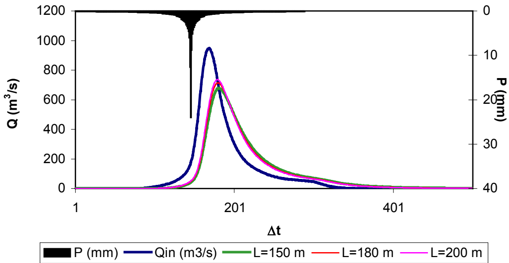
FIGURA 8.1 – HIDROGRAMAS DE ENTRADA E DE SAÍDA DO RESERVATÓRIO RIACHO DO MEIO (TR=1.000 ANOS, PERFIL CREAGER)
