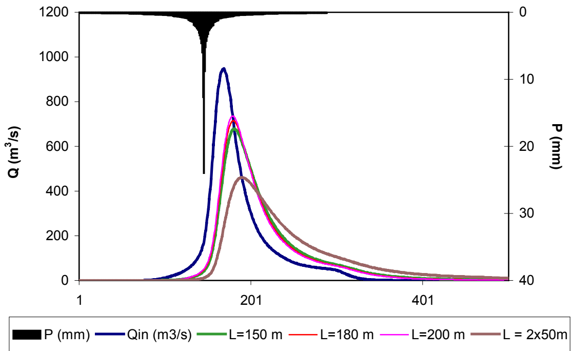
FIGURA 8.5 – HIDROGRAMAS DE ENTRADA E DE SAÍDA DO RESERVATÓRIO RIACHO DO MEIO (TR=1.000 ANOS, PERFIL CREAGER)
