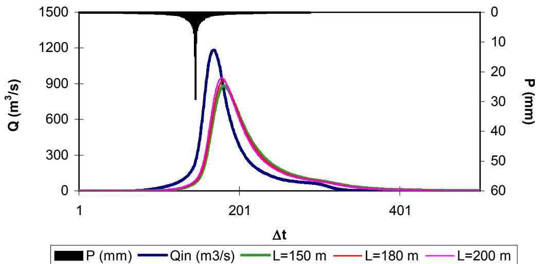
FIGURA 8.2 – HIDROGRAMAS DE ENTRADA E DE SAÍDA DO RESERVATÓRIO RIACHO DO MEIO (TR=10.000 ANOS, PERFIL CREAGER)
