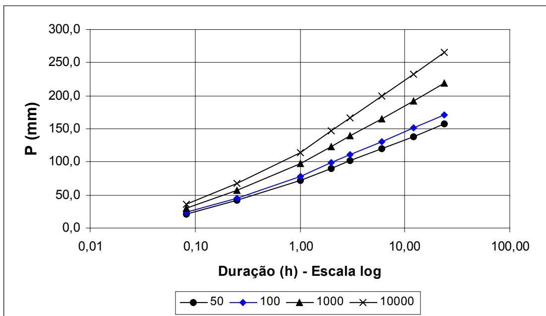
FIGURA 6.1 – CURVAS INTENSIDADE-DURAÇÃO-FREQÜÊNCIA - CHUVA REDUZIDA
