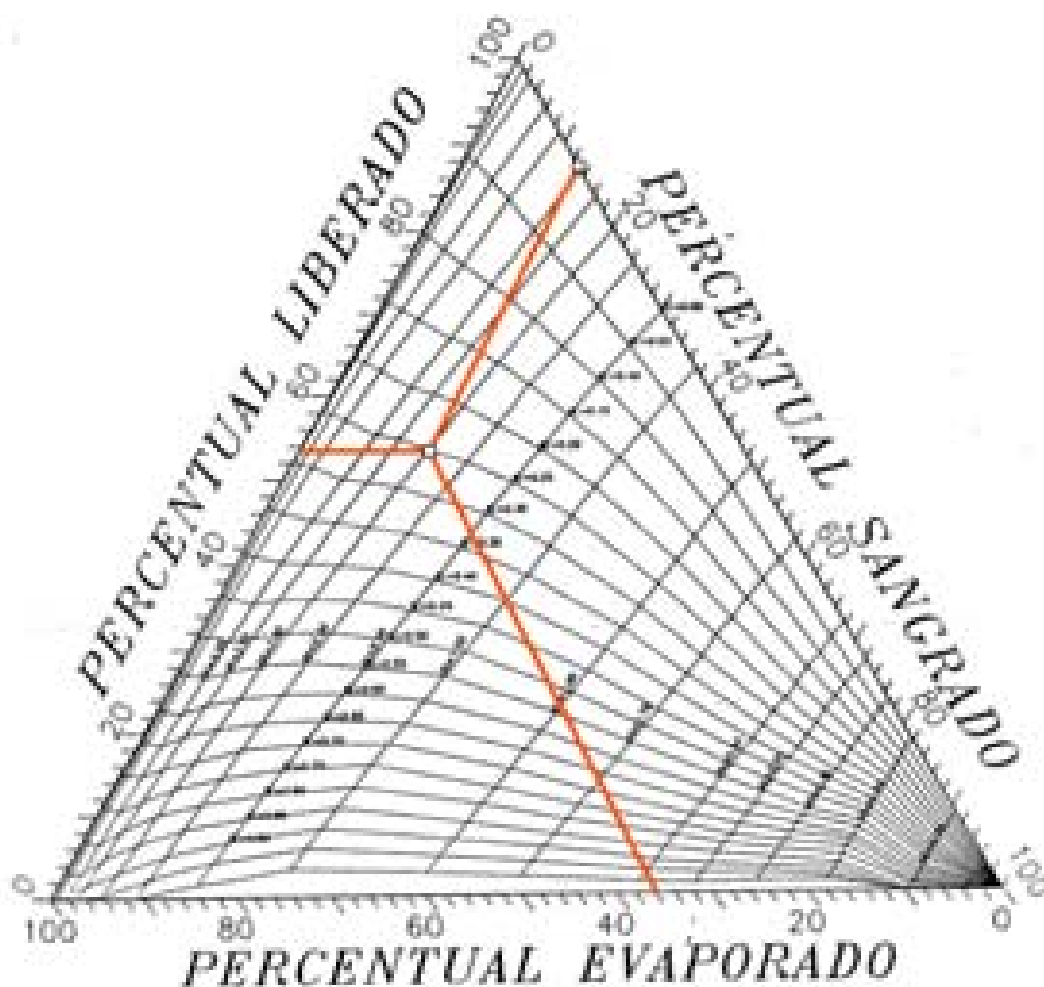
FIGURA 7.2 – DIAGRAMA TRIANGULAR DE REGULARIZAÇÃO APLICADO A BARRAGEM RIACHO DO MEIO.
