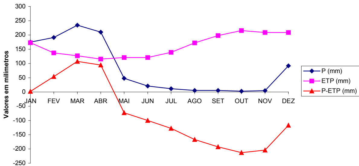
FIGURA 4.5 – BALANÇO HÍDRICO
