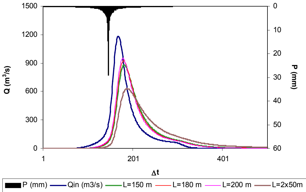
FIGURA 8.6 – HIDROGRAMAS DE ENTRADA E DE SAIDA DO RESERVATÓRIO RIACHO DO MEIO (TR=10.000 ANOS, PERFIL CREAGER).
