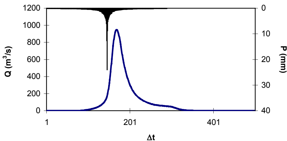
FIGURA 6.2 – HIDROGRAMA TOTAL AFLUENTE AO RIACHO DO MEIO (TR = 1000 ANOS)
