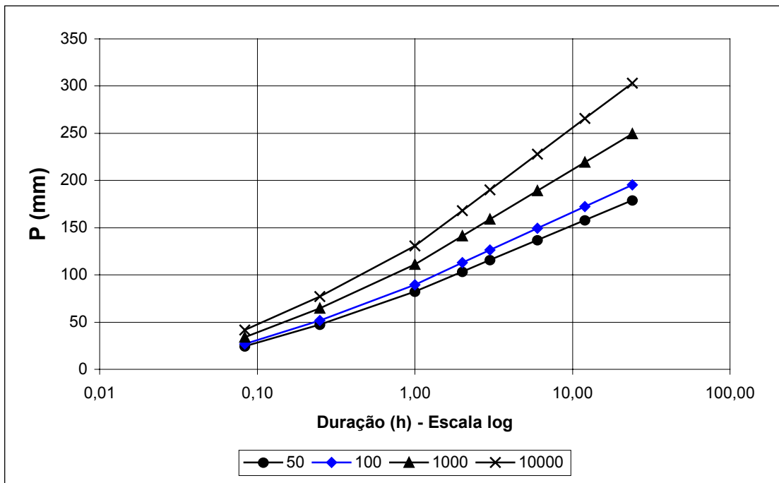
FIGURA 5.4 – CURVAS INTENSIDADE-DURAÇÃO-FREQUÊNCIA
