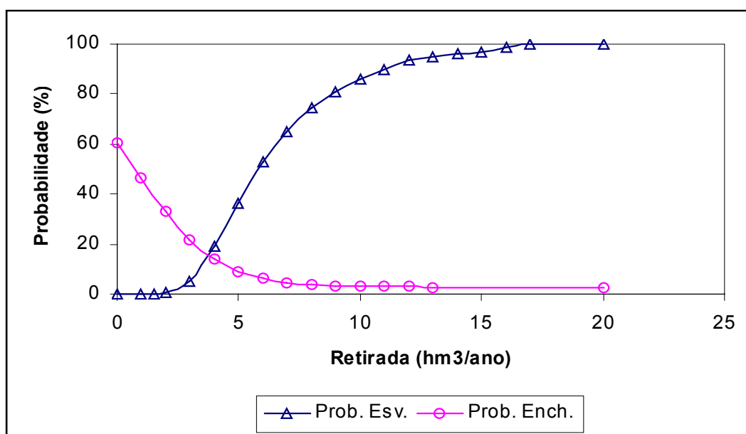
FIGURA 10.1 – PROBABILIDADES DE ESVAZIAMENTO E ENCHIMENTO DO AÇUDE RIACHO DO MEIO
