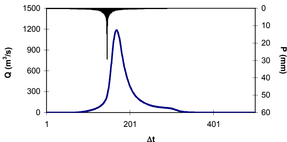
FIGURA 6.3 – HIDROGRAMA TOTAL AFLUENTE AO RIACHO DO MEIO (TR = 10000 ANOS)
