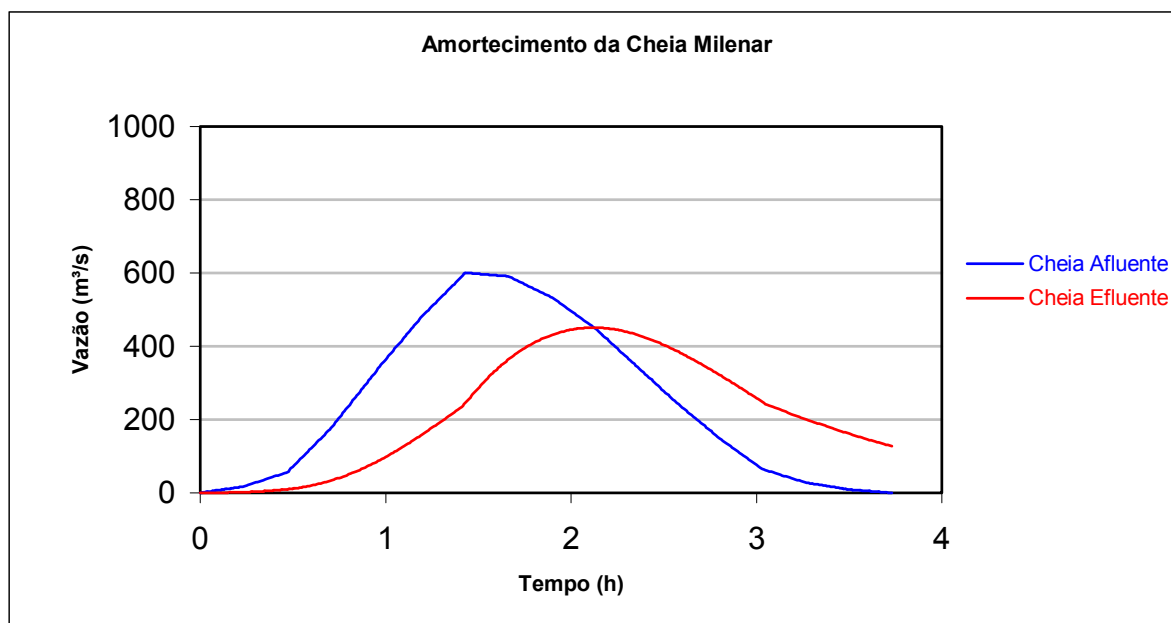
FIGURA 8.1 – Amortecimento da cheia milenar para cotas do sangradouro do Açude Retirana
