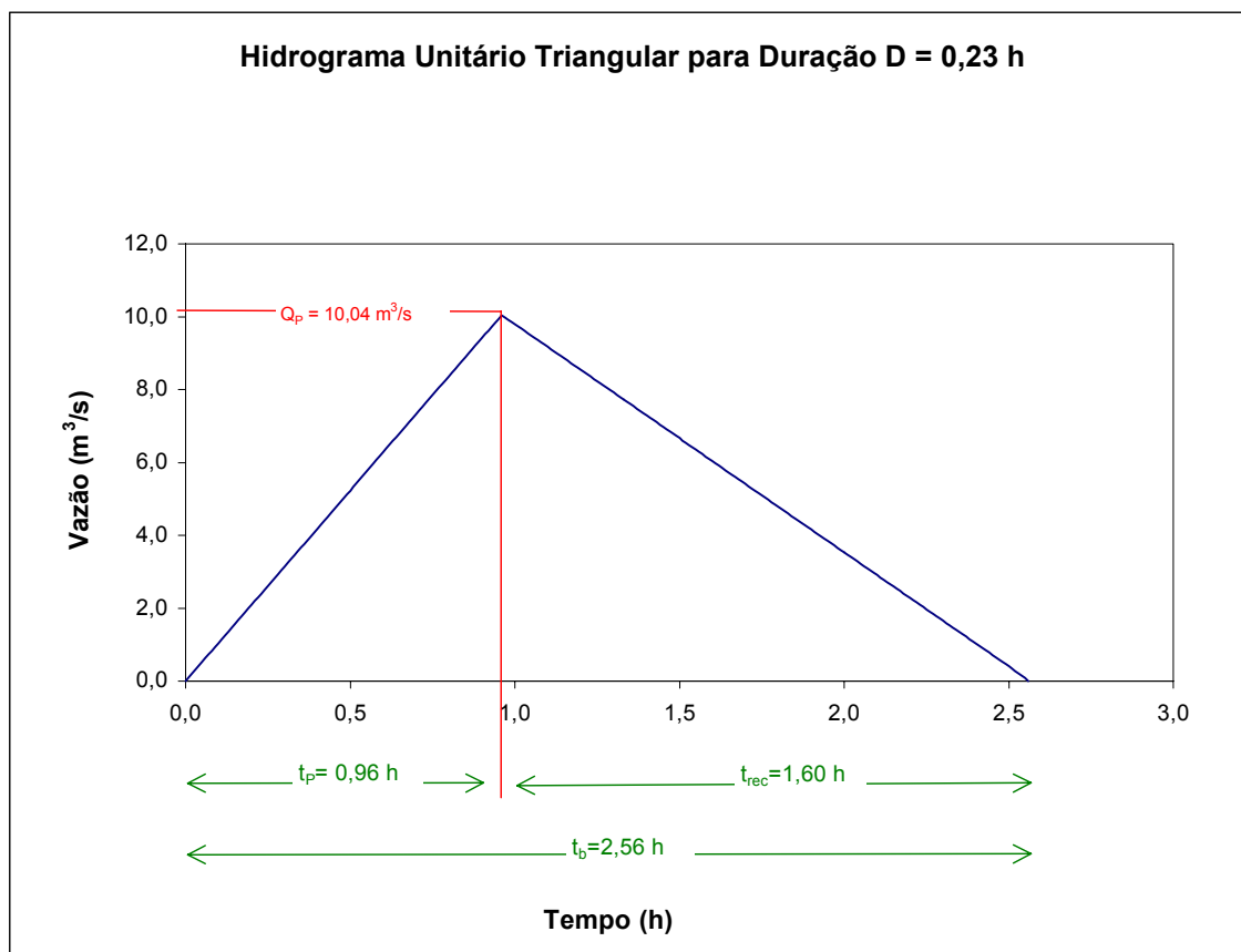
Figura 6.2 - Hidrograma unitário triangular do SCS para duração de 0,23 horas
