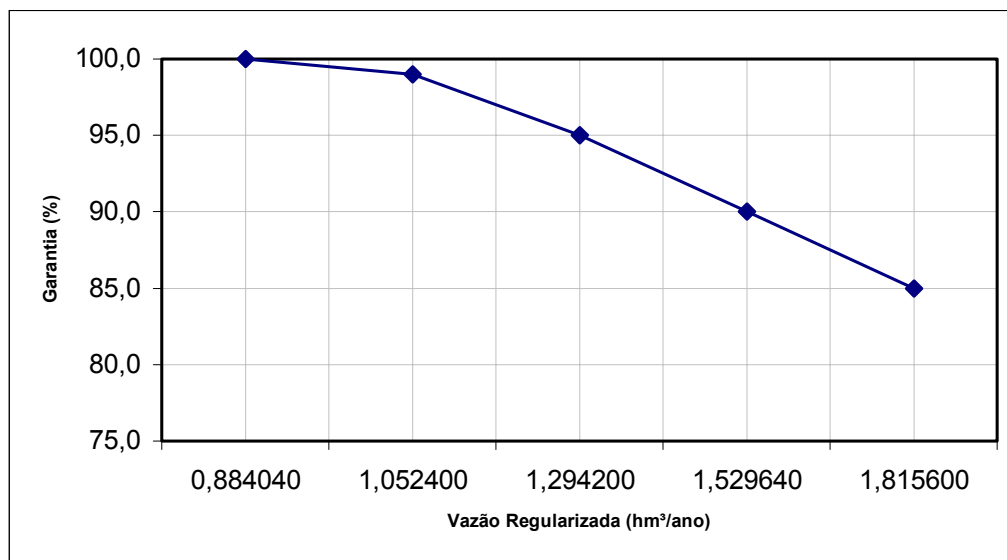
Figura 6.1 – Curva Garantia versus Vazão Regularizada do açude Retirana, para a Capacidade de 5,898hm 3 (cota = 473,0 m ).
