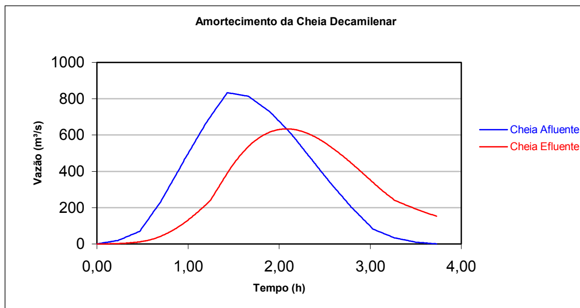
FIGURA 8.2 – Amortecimento da cheia decamilenar para cotas do sangradouro do Açude Retirana
