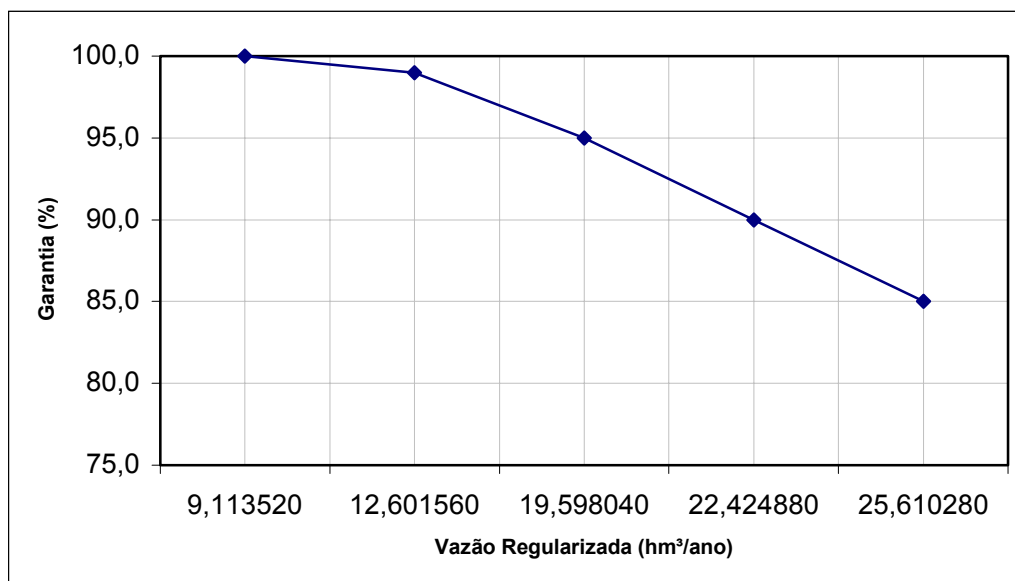
Figura 6.1 - Curva Garantia versus Vazão Regularizada do açude Raízes, para a Capacidade de 12,766 hm 3 (cota = 14,5 m ).
