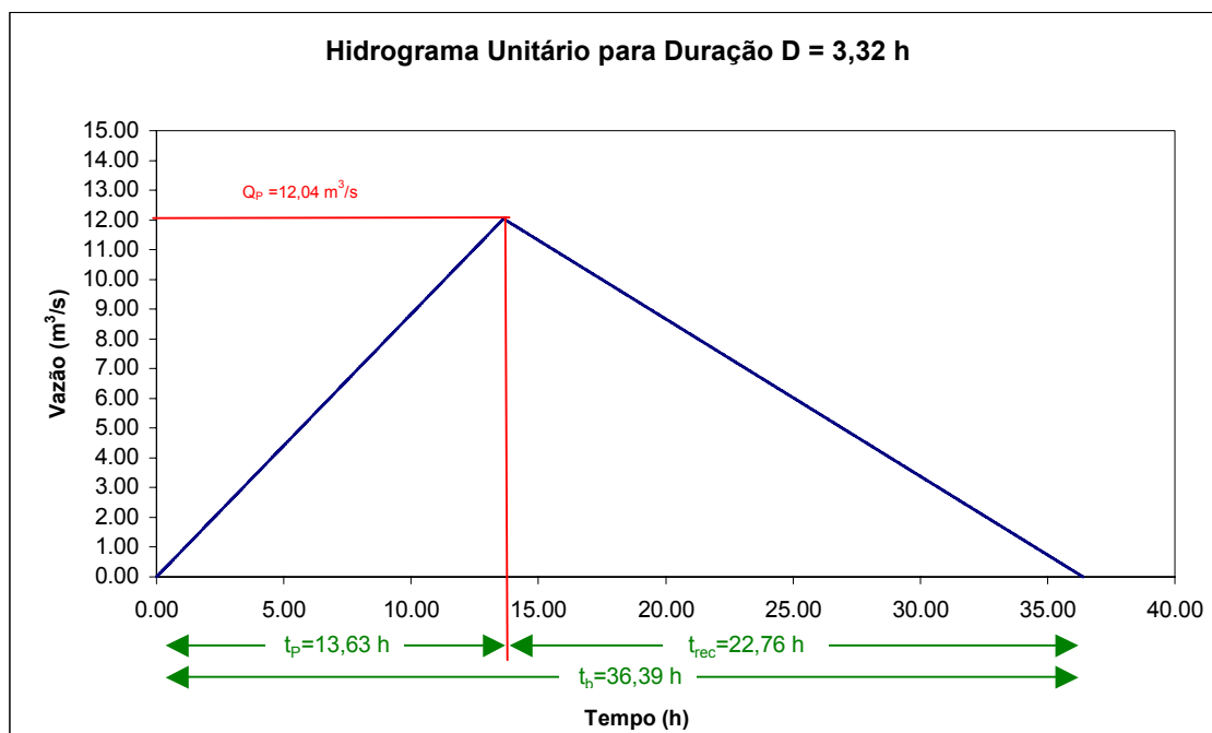
Figura 6.2 - Hidrograma unitário triangular do SCS para duração de 3,32 horas
