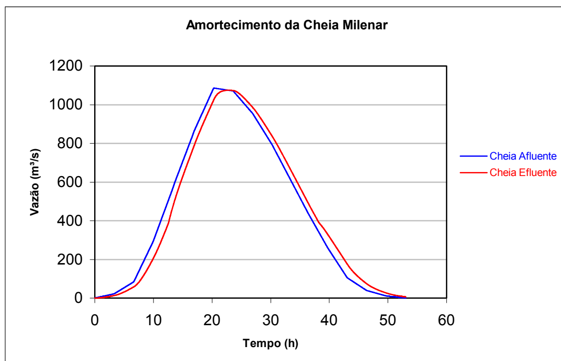
FIGURA 8.1 - Amortecimento da cheia milenar para cotas do vertedouro do Açude Raízes
