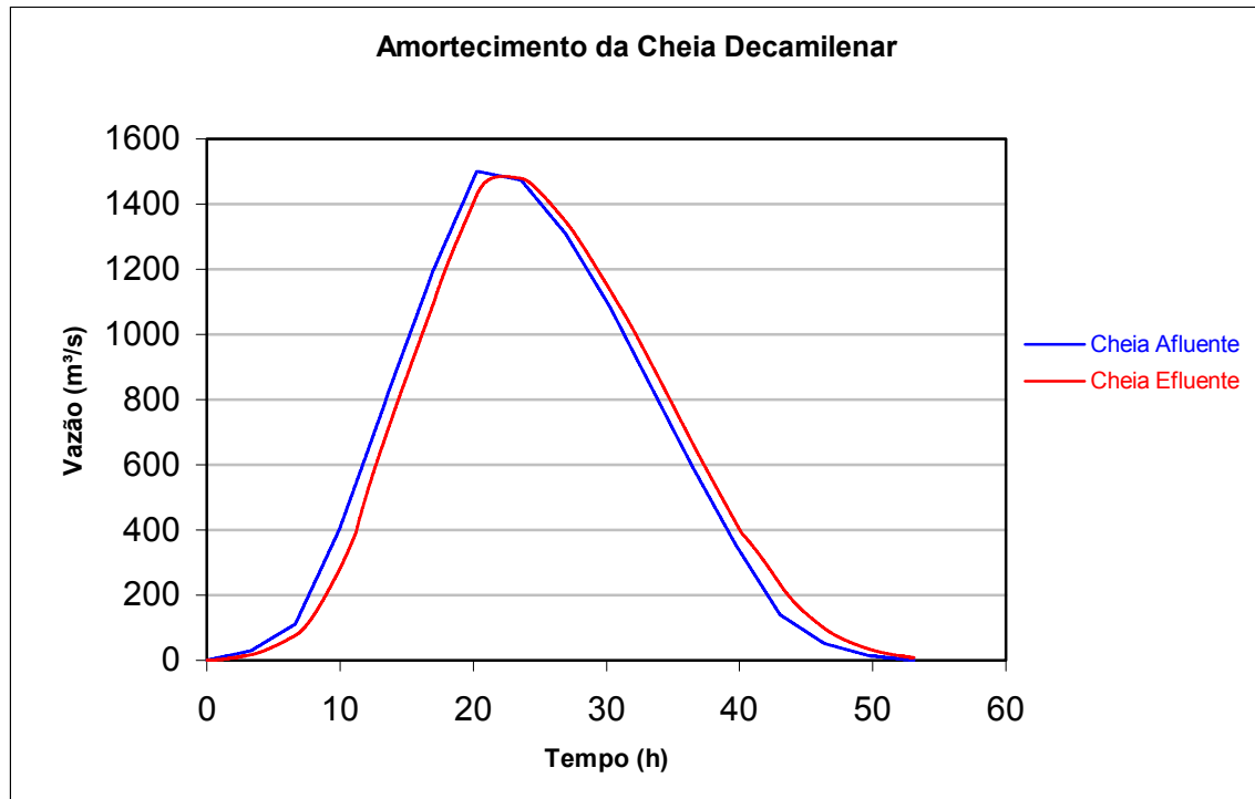
FIGURA 8.2 - Amortecimento da cheia decamilenar para cotas do vertedouro do Açude Raízes
