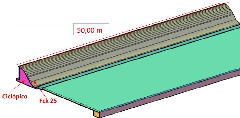
SEÇÃO DO CREAGER
