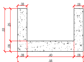
FORMA DA CALHA (TALUDE, BERMA E OMBREIRA) ESCALA - 1:10
