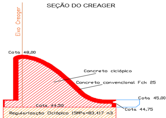
SEÇÃO DO CREAGER
