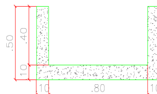
CORTE - CC FORMA ESCALA - 1:25
