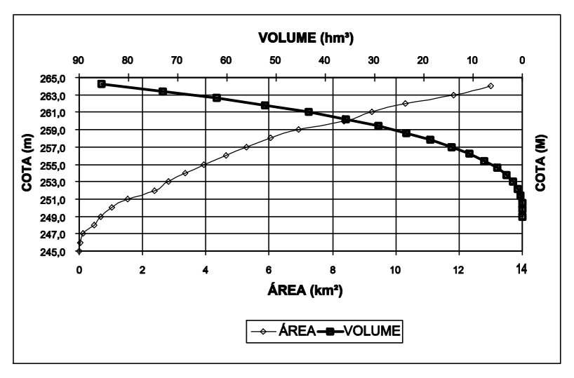
CURVA COTA x ÁREA x VOLUME
