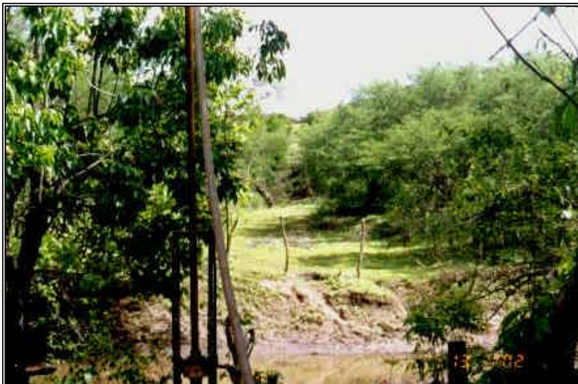
FOTO 03 – EIXO SUL DA BARRAGEM A SER CONSTRUÍDA.
