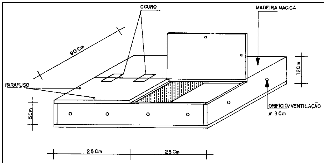
Figura 9.5 - Caixa para Transporte de Ofídios - Modelo Butantã
