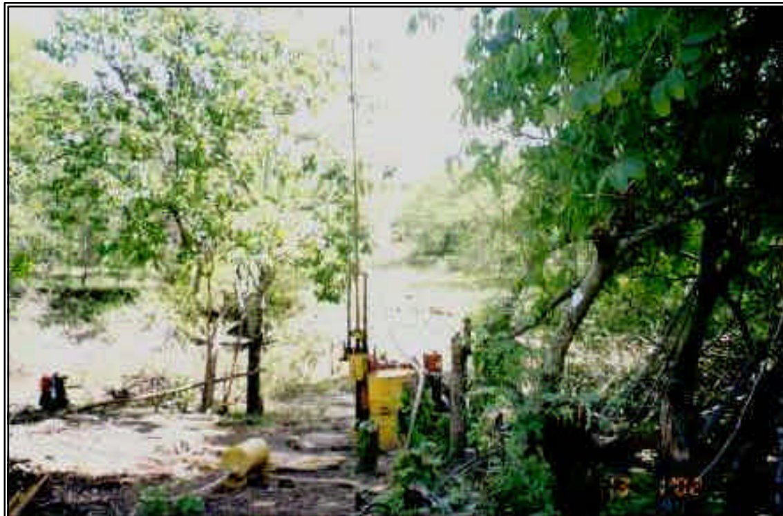
FOTO 02 – EIXO DA BARRAGEM E EQUIPAMENTO DE PROSPECÇÃO GEOLÓGICA.
