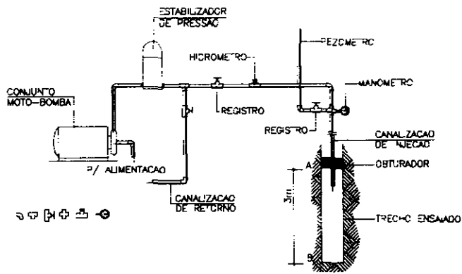
EQUIPAMENTO PARA ENSAIO DE PERDA D'AGUA (LUGEDN)
